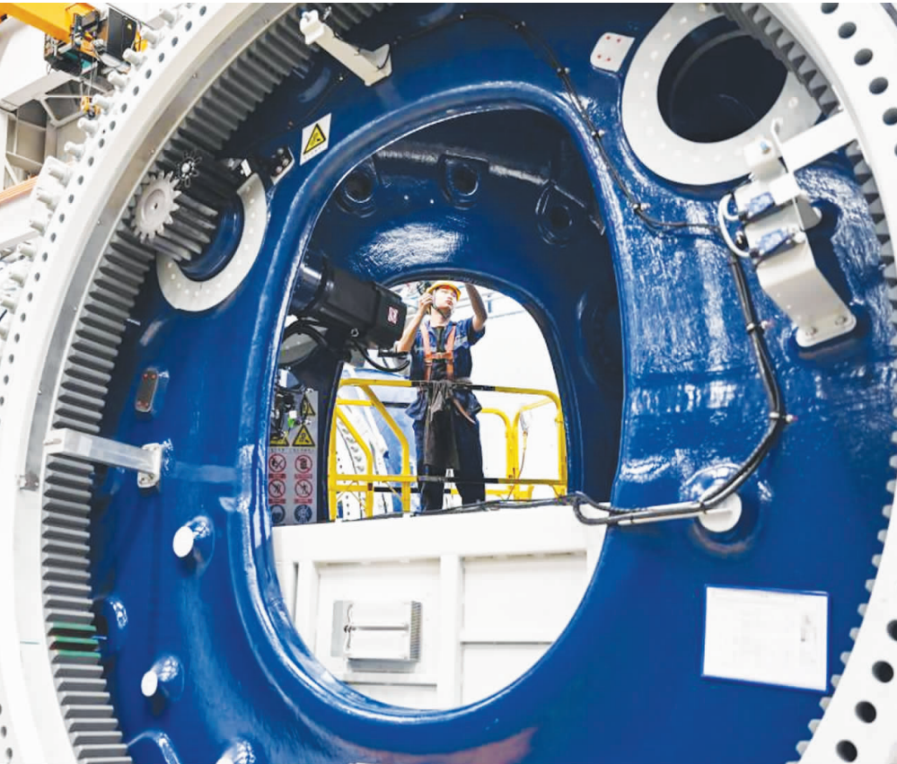
工人在包头市明阳新能源智能制造产业园总装车间作业 李志鹏 摄
