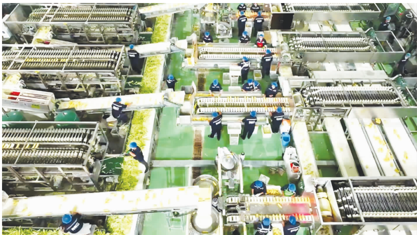
鲜食玉米加工流水线
